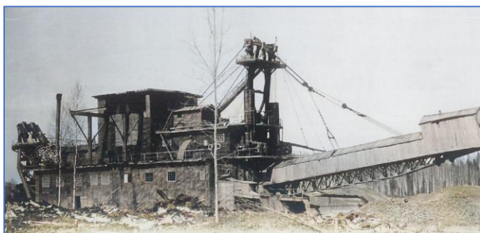
Драга №29 (черная) на реке Выя. 1944г.
