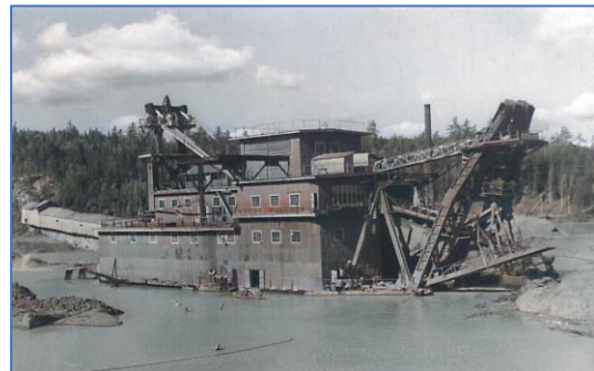
Драга №25 на реке Ис
